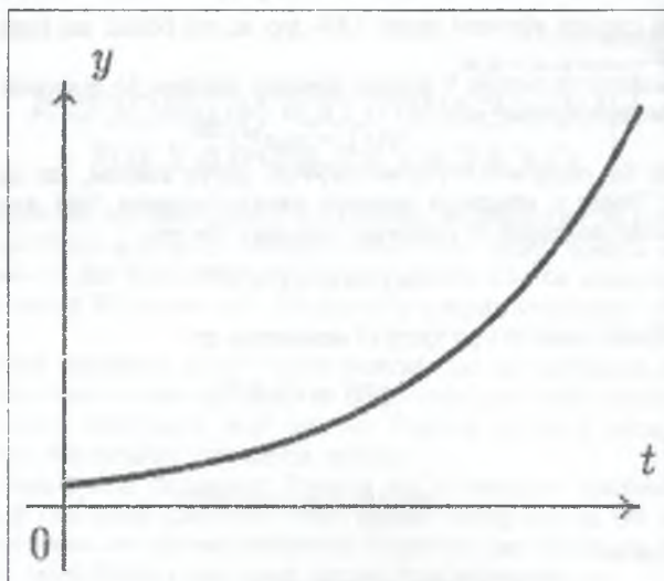
Расми 1. Графики функцияи y = Ce^{kx}
